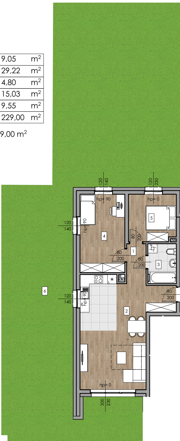
BUDYNEK B / PARTER / MIESZKANIE B0_01
